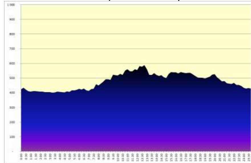
Tipikus munkaszüneti napi terhelési diagram 2015. szeptember 6. vasárnap
