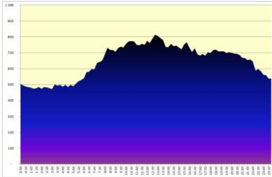
Tipikus munkanapi terhelési diagram 2015. március 11. szerda
