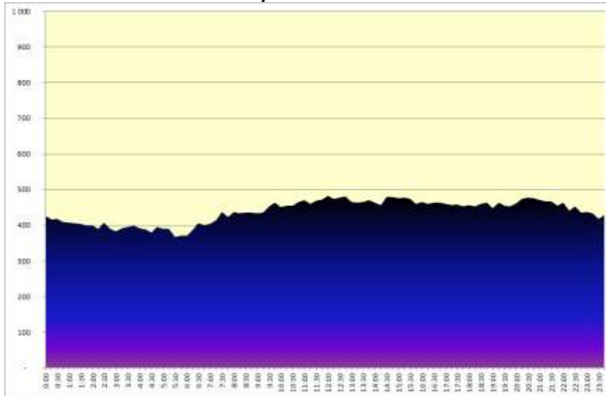
Tipikus szabadnapi terhelési diagram 2015. április 25. szombat
