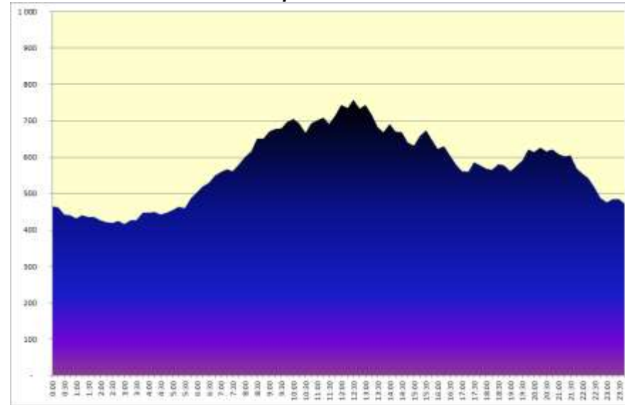
Tipikus munkanapi terhelési diagram 2015. szeptember 9. szerda
